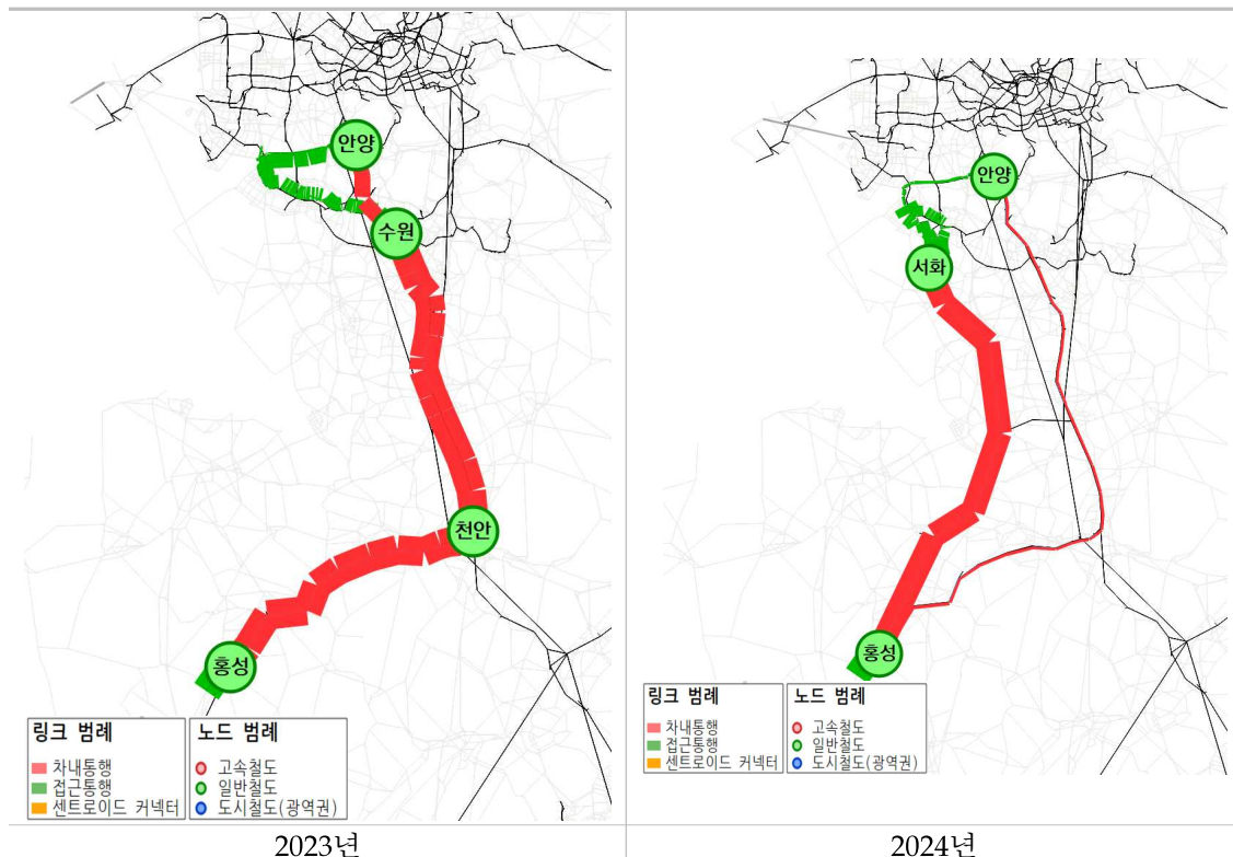
〈그림 6-11〉 기준연도 일반철도 통행시간/거리 검증(홍성-시흥)
