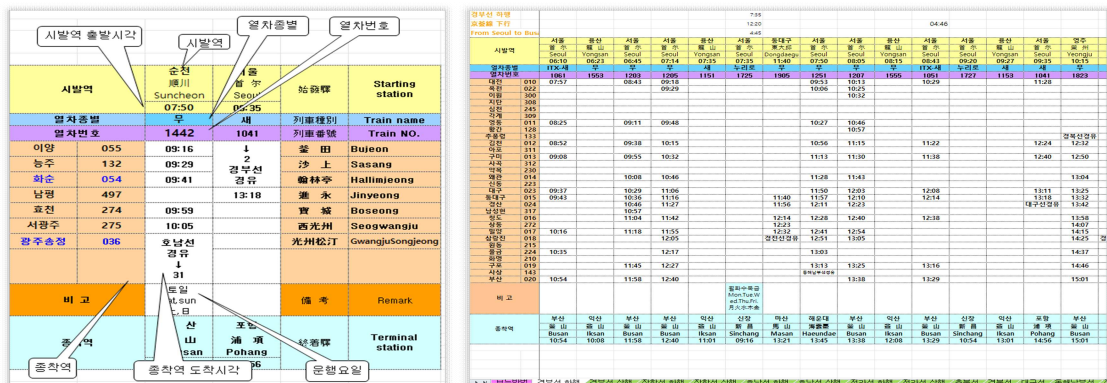
〈그림 2-5〉 일반철도 시각표 구성 및 시각표테이블 예시
